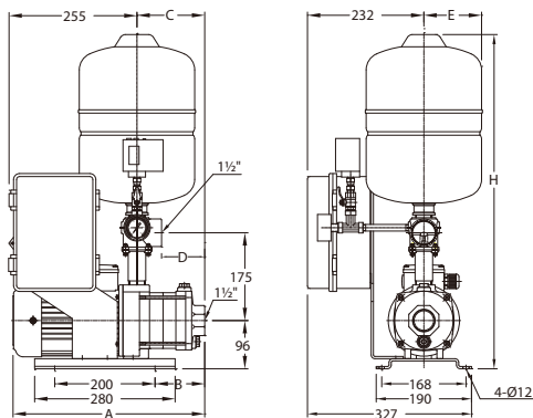
外型尺寸 TPH4T X (mm)
