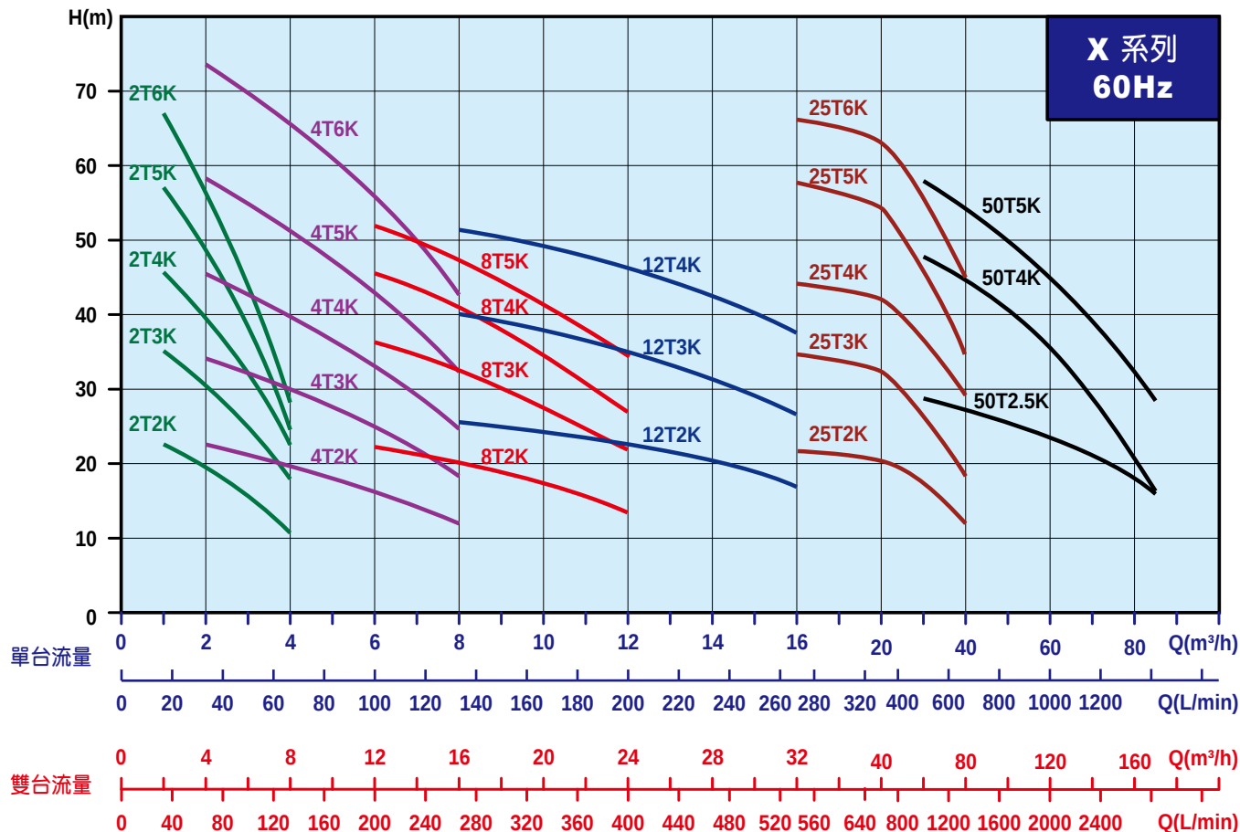
特性曲線
