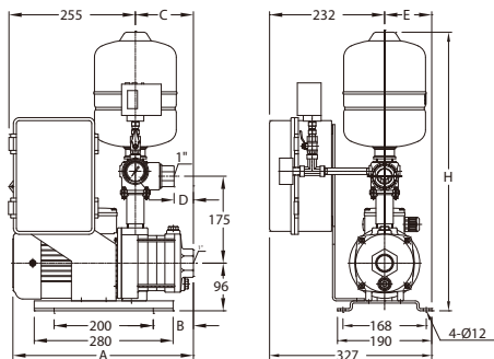
外型尺寸 TPH2T X (mm)
